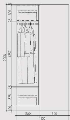
ELEVATION A
